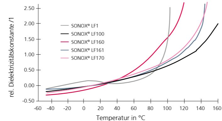
Relative Temperaturabhängigkeit der Dielektrizitätskonstante
